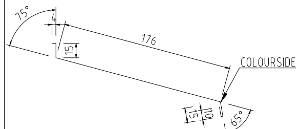
UNDERBLECK FÖNSTER 170 Tj=0,6 L=1200, 1500, 2000mm KB=220mm
