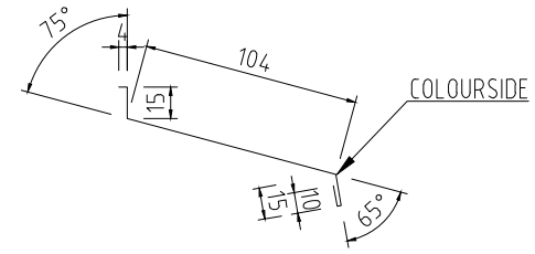
UNDERBLECK FÖNSTER 100 Tj=0,6 L=1200, 1500, 2000mm KB=148mm
