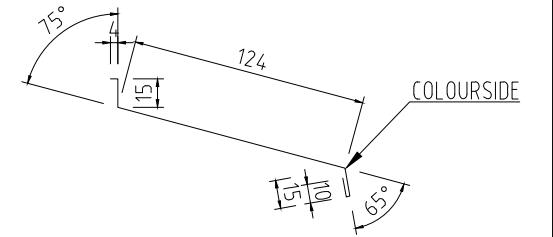
UNDERBLECK FÖNSTER 120 Tj=0,6 L=1200, 1500, 2000mm KB=168mm
