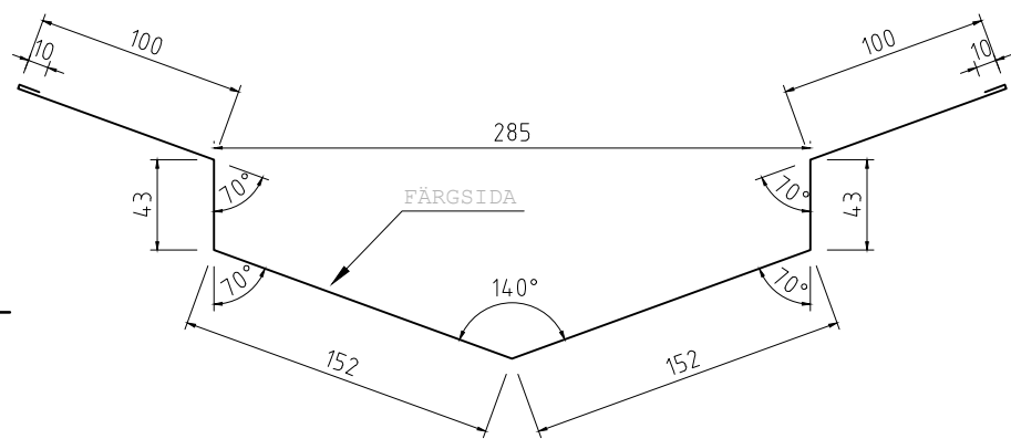
RÄNNDALSPLÅT KNÄCKT 152x152 Tj=0,5-0,6 L=2000mm KB=610mm
