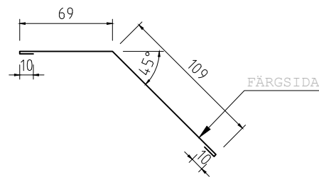
FOTPLÅT 69x109 VÄNDBAR Tj=0,5-0,6 L=2000mm KB=198mm
