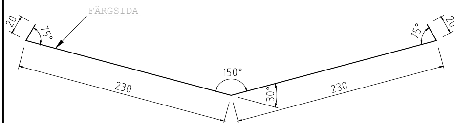
RÄNNDALSPLÅT RAK 230x230 Tj=0,5-0,6 L=2000mm KB=500mm
