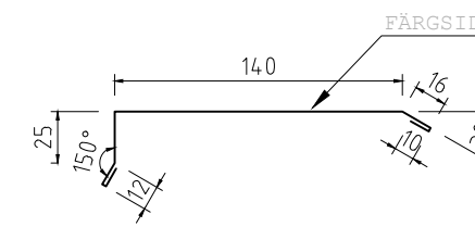
GAVELBESLAG RAK 25x140 Tj=0,5-0,6 L=2000mm KB=213mm
