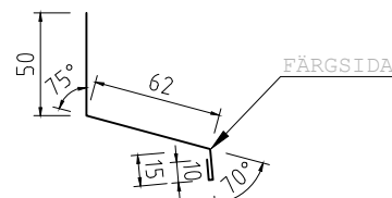
ÖVERBLECK FÖNSTER 60 Tj=0,6 L=1200, 1500, 2000mm KB=137mm
