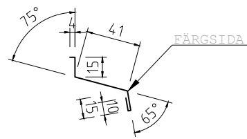
UNDERBLECK FÖNSTER 40 Tj=0,6 L=1200, 1500, 2000mm KB=85mm
