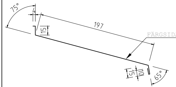
UNDERBLECK FÖNSTER 190 Tj=0,6 L=1200, 1500, 2000mm KB=241mm
