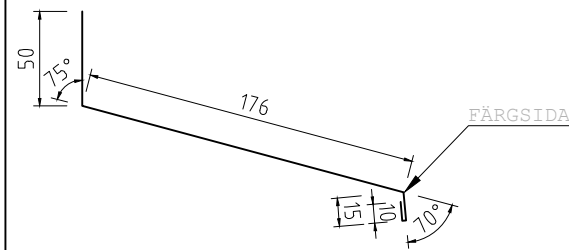
ÖVERBLECK FÖNSTER 170 Tj=0,6 L=1200, 1500, 2000mm KB=251mm
