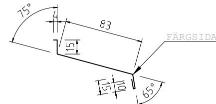
UNDERBLECK FÖNSTER 80 Tj=0,6 L=1200, 1500, 2000mm KB=127mm
