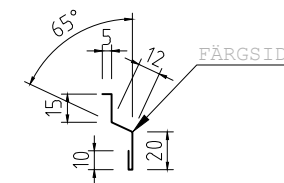
TRÖSKELBLECK 1230 Tj=0,5-0,6 L=1230mm KB=62mm
