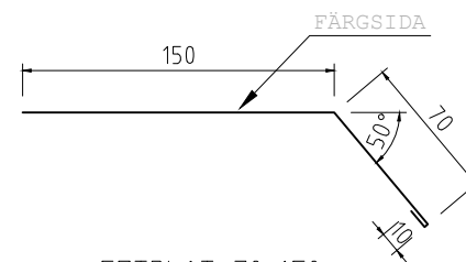
FOTPLÅT 70x150 Tj=0,5-0,6 L=2000mm KB=230mm
