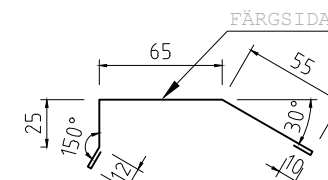
GAVELBESLAG KNÄCKT 25x65x55 Tj=0,5-0,6 L=2000mm KB=177mm
