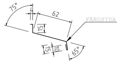
UNDERBLECK FÖNSTER 60 Tj=0,6 L=1200, 1500, 2000mm KB=106mm
