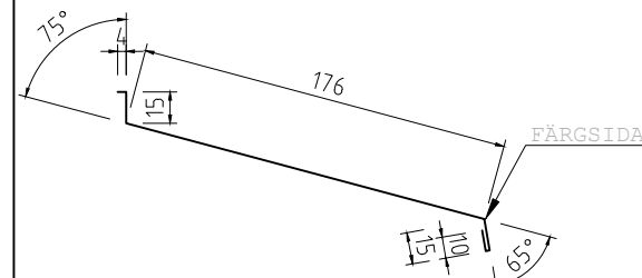
UNDERBLECK FÖNSTER 170 Tj=0,6 L=1200, 1500, 2000mm KB=220mm
