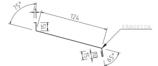
UNDERBLECK FÖNSTER 120 Tj=0,6 L=1200, 1500, 2000mm KB=168mm
