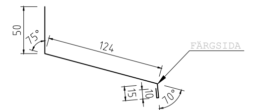
ÖVERBLECK FÖNSTER 120 Tj=0,6 L=1200, 1500, 2000mm KB=199mm
