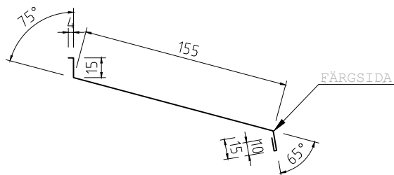
UNDERBLECK FÖNSTER 150 Tj=0,6 L=1200, 1500, 2000mm KB=199mm
