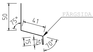
ÖVERBLECK FÖNSTER 40 Tj=0,6 L=1200, 1500, 2000mm KB=116mm
