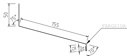
ÖVERBLECK FÖNSTER 150 Tj=0,6 L=1200, 1500, 2000mm KB=230mm
