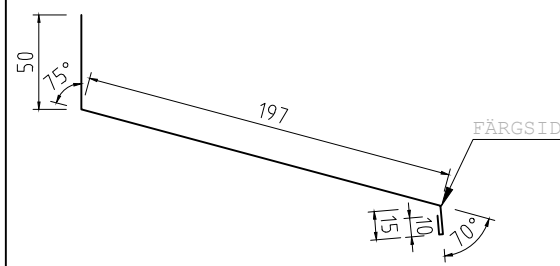
ÖVERBLECK FÖNSTER 190 Tj=0,6 L=1200, 1500, 2000mm KB=272mm
