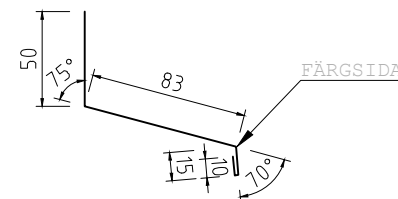
ÖVERBLECK FÖNSTER 80 Tj=0,6 L=1200, 1500, 2000mm KB=158mm
