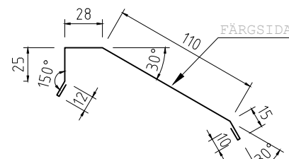
GAVELBESLAG KNÄCKT 25x28x110 Tj=0,5-0,6 L=2000mm KB=210mm
