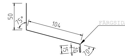
ÖVERBLECK FÖNSTER 100 Tj=0,6 L=1200, 1500, 2000mm KB=179mm
