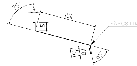
UNDERBLECK FÖNSTER 100 Tj=0,6 L=1200, 1500, 2000mm KB=148mm
